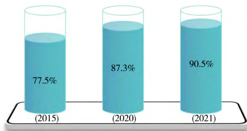
图2 2015、2020、2021年地表水国考断面水质优良率
