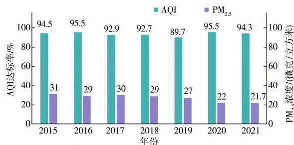
图1 2015—2021年AQI达标率和PM 2.5 浓度
